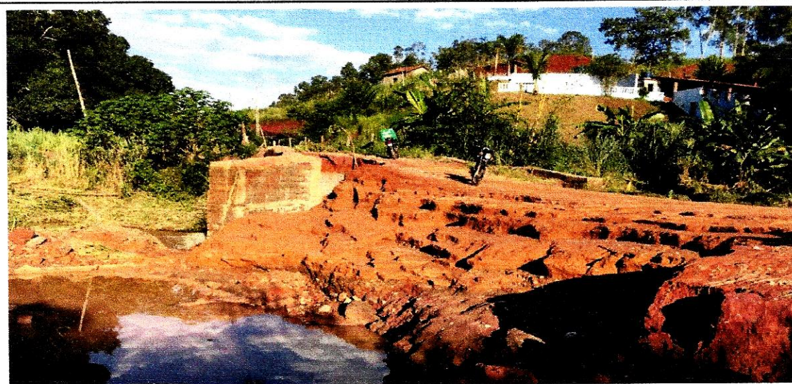
Ponte Gumercino Gomes de Freitas, localizada no Córrego dos Barbosas e Elias. Santa Maria, Zona Rural de Visconde do Rio Branco - MG
